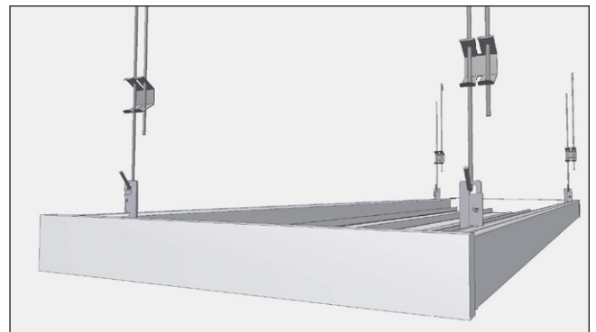
Figur 8. Atrium frithængende i justerbare pendler i kombination med Atrium panelkroge.
