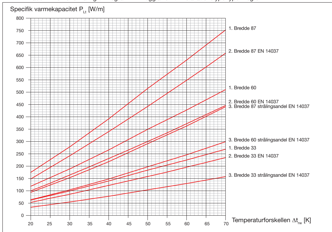
Diagram 1. Atrium-H og Loggia, specifik varmekapacitet P_{Lt} pr. aktiv længde ved nominal vandmængde i en varmestrips med q_{wnom} = 0,011 \text{ l/s} .
