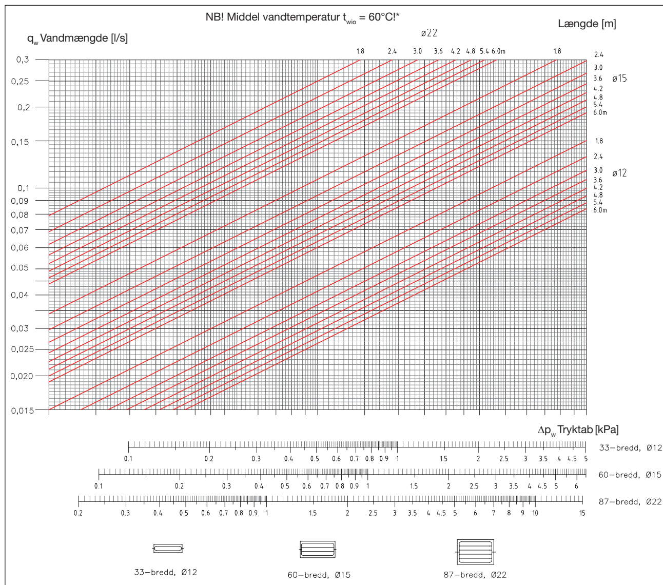
Diagram 5. Paneler, tryktab ved temperatur 60^\circ\text{C} . For tryktab ved andre temperaturer end 60^\circ\text{C} , multipliceres tryktabet med tryktabsfaktoren (se diagram 7).
