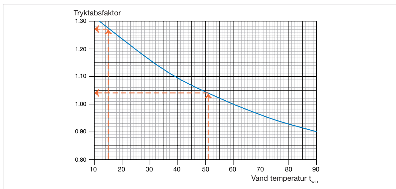
Diagram 7. Temperaturkorrigeret tryktabsfaktor.
