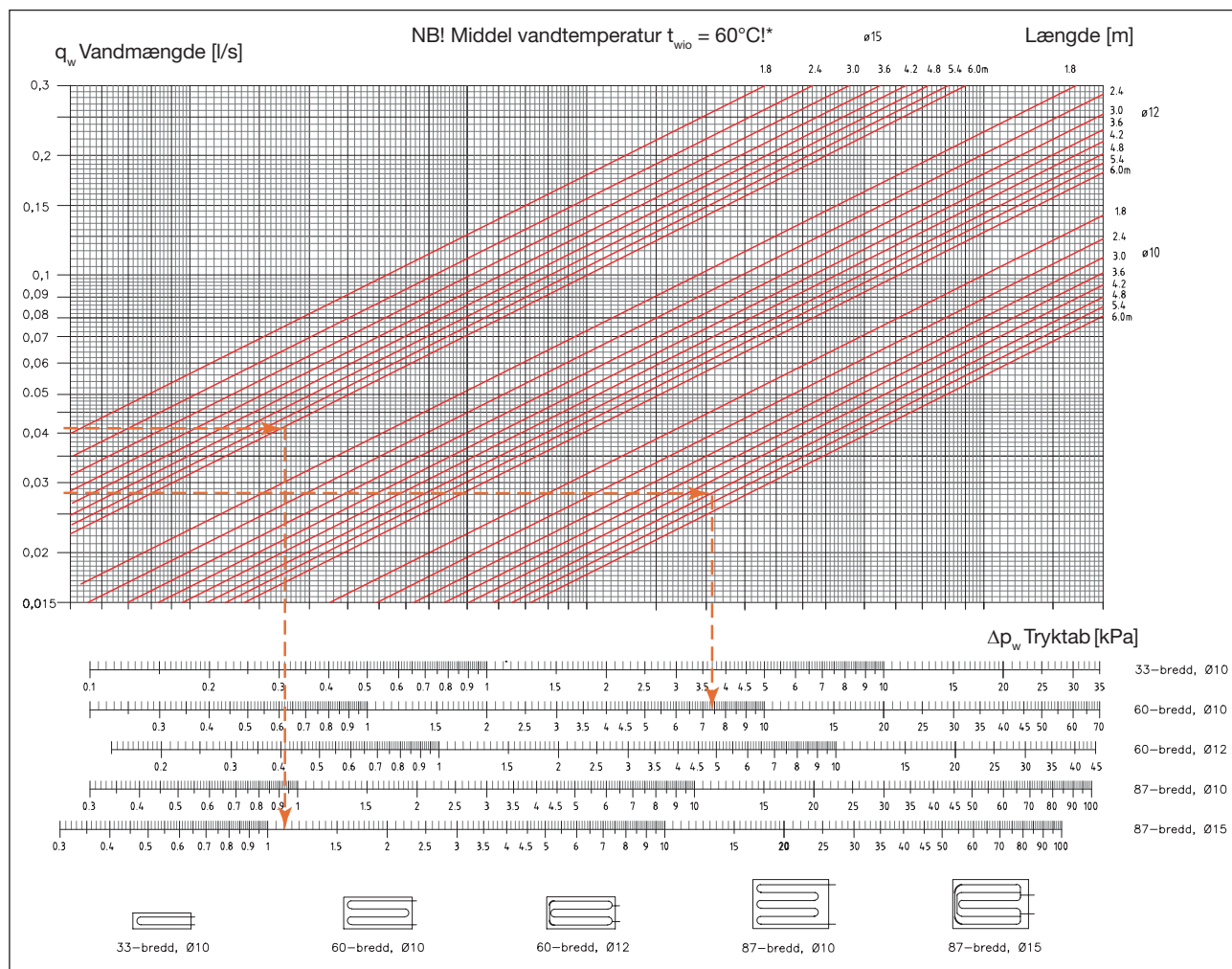
Diagram 4. Paneler, tryktab ved temperatur 60°C. For tryktab ved andre temperaturer end 60°C, multipliceres tryktabet med tryktafsfaktoren (se diagram 7).
